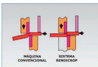
Система предотвращения деформации типа искривления при резке полосы
